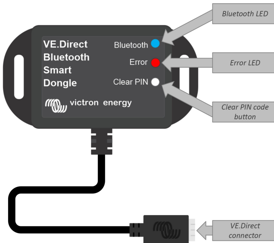
Emplacement des LED, du bouton PIN et du connecteur VE.Direct sur la clé électronique VE.Direct Bluetooth Smart.
