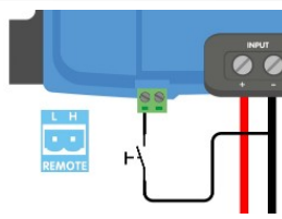
c) Câblage de la broche L
